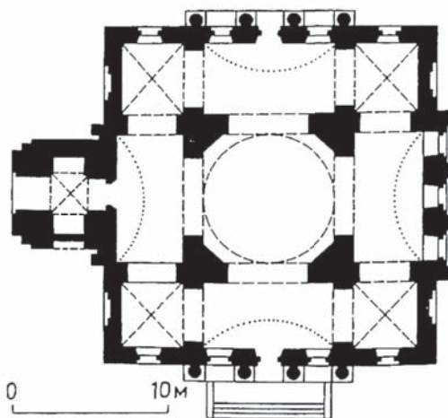
План храма Рождества Христова в селе Рождествено. Из книги «Памятники архитектуры Московской области»
